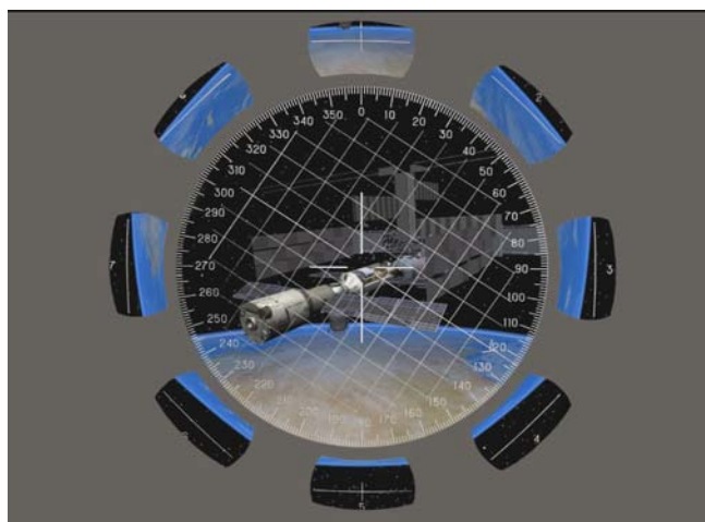
Рис. 2 Имитация прибора контроля за ориентацией космического аппарата
