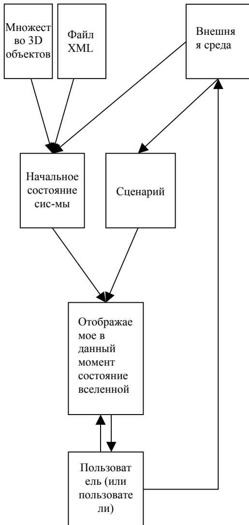
Рис 1. Существующая схема работы приложения
