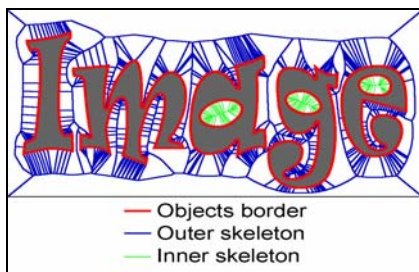
Рис. 1. Непрерывное гранично-скелетное представление изображения.
