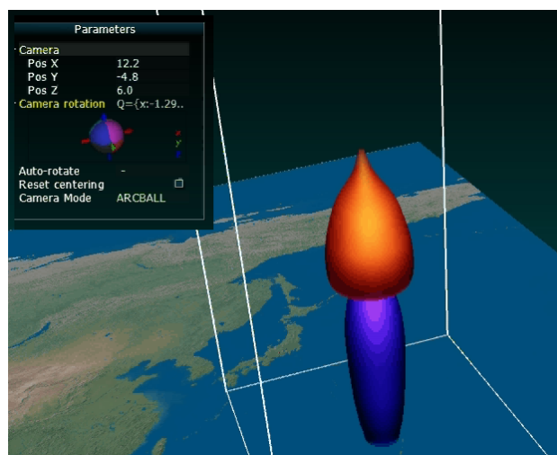
Рис. 4: Визуализация температурных аномалий в ядре тропического циклона.
