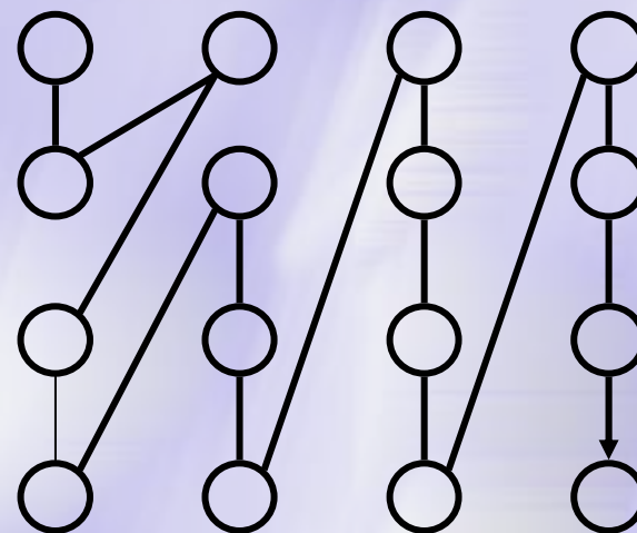
intra 4x4 для interlaced video
